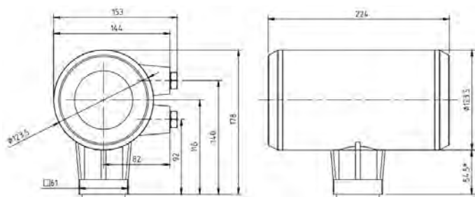
Исполнение 1 (стандартный ЭБ)
