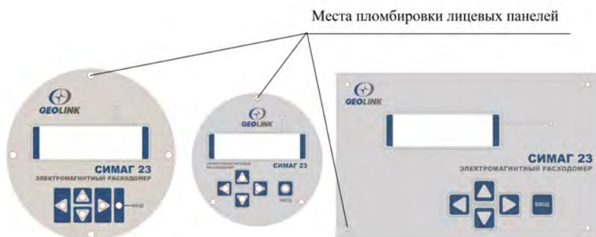
Рисунок 10.3 – Места пломбировки лицевых панели электронного блока
