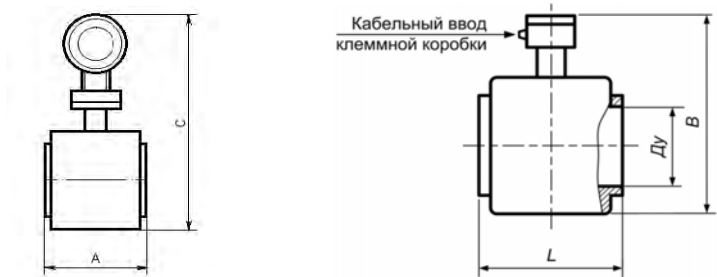
Рисунок Б.5 – Конструкция сенсора без фланцев ("Сэндвич")
