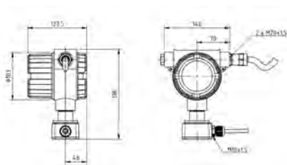
Исполнение 2 (малогобаритный ЭБ)
